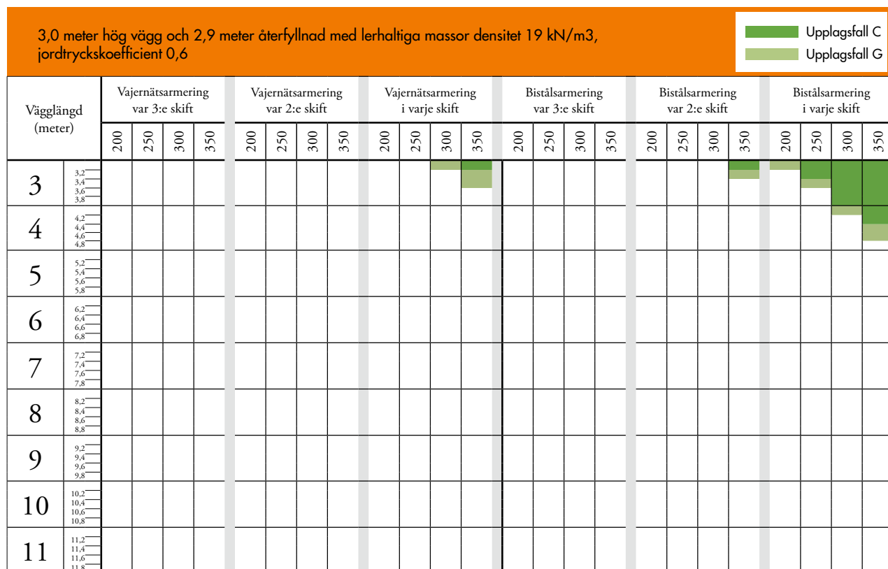
Diagram 2.8 Högsta tillåtna vägg längd mellan stödvägg på 3,0 m hög källarvägg återfylld med 2,9 m lerhaltiga massor vid olika armeringsintervall och blockstorlek.
