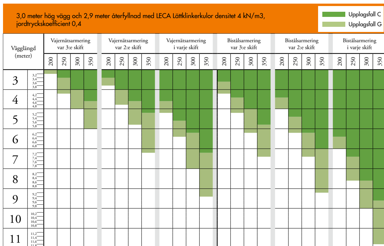
Diagram 2.9 Högsta tillåtna vägg längd mellan stödvägg på 3,0 m hög källarvägg återfylld med 2,9 m LECA Lättklinkerkulor vid olika armeringsintervall och blockstorlek.
