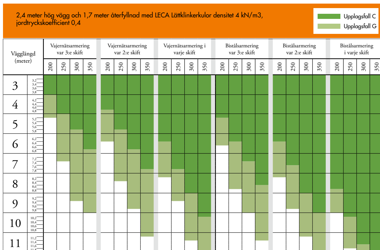
Diagram 2.3 Högsta tillåtna vägglängd mellan stödväggar på 2,4 m hög källarvägg återfylld med 1,7 m LECA Lättklinkerkulor vid olika armeringsintervall och blockstorlek.
