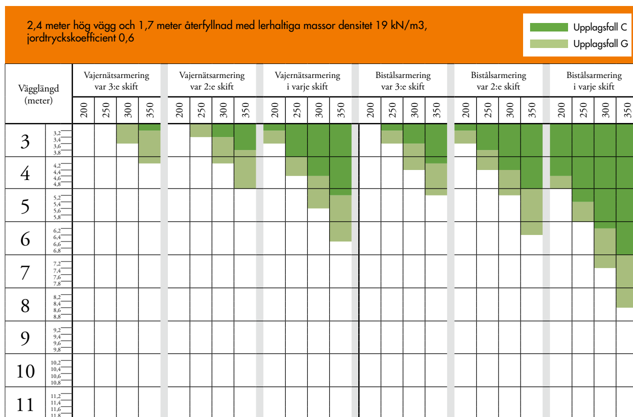
Diagram 2.2 Högsta tillåtna vägglängd mellan stödväggar på 2,4 m hög källarvägg återfylld med 1,7 m lerhaltiga massor vid olika armeringsintervall och blockstorlek.
