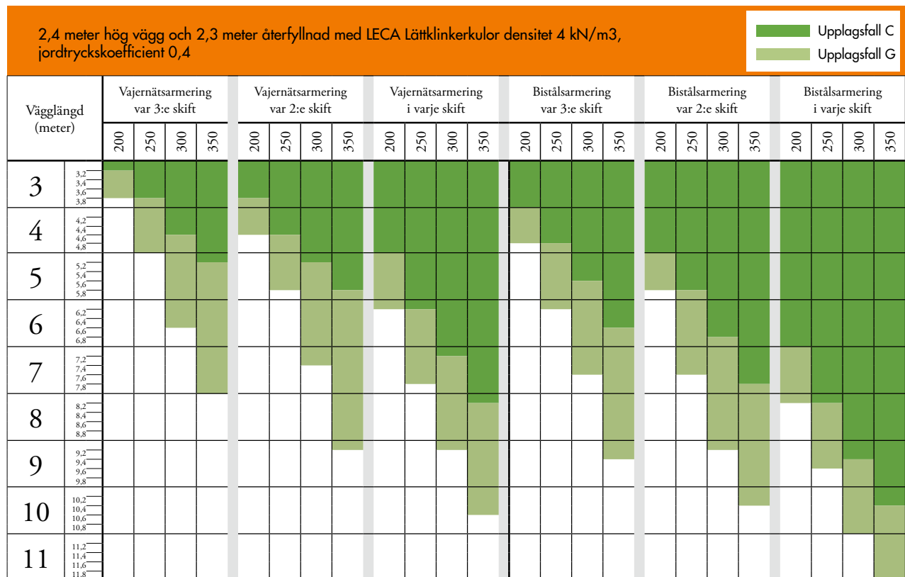
Diagram 2.6 Högsta tillåtna vägglängd mellan stödväggar på 2,4 m hög källarvägg återfylld med 2,3 m LECA Lättklinkerkulor vid olika armeringsintervall och blockstorlek.
