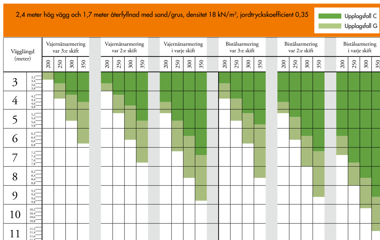
Diagram 2.1 Högsta tillåtna väggglängd mellan stödväggar på 2,4 m hög källarvägg återfylld med 1,7 m sand/grus vid olika armeringsintervall och blockstorlek.
