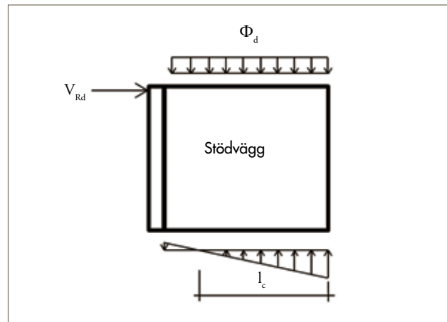
Bild 3.7. Krafter som verkar på stödväggen.
