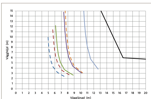
Diagram 3.7 Maximal väggstorlek för LECA block 300 med 1,2 kN/m 2 vindlast och upplag A.
