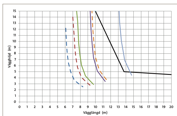
Diagram 3.11 Maximal väggstorlek för LECA block 250 med 1,2 kN/m 2 vindlast och upplag C.
