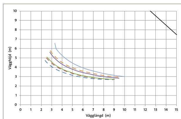
Diagram 3.26 Maximal väggstorlek för LECA block 250 med 1,2 kN/m 2 vindlast och upplag J.
