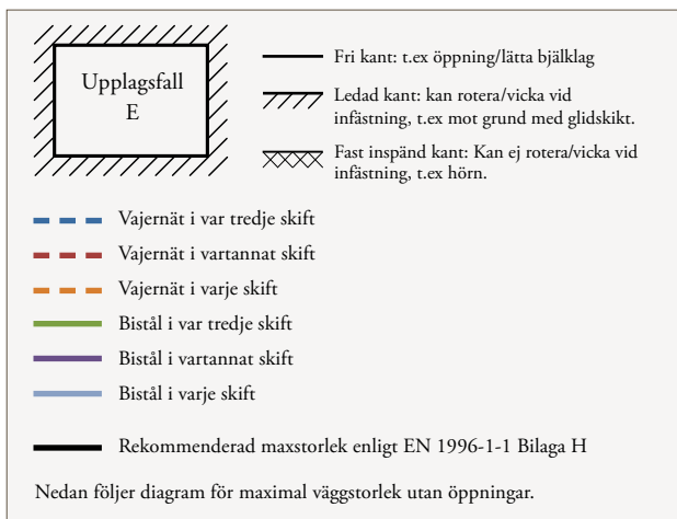
Diagram 3.16 Maximal väggstorlek för LECA block 250 med 1,2 kN/m 2 vindlast och upplag E.
