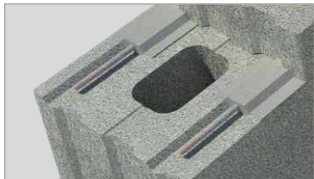
Bild 3.4 Ringarmering.
