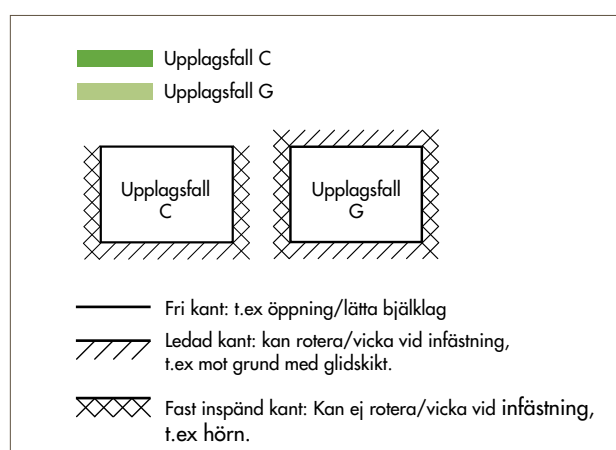
Bild 2.7 Upplagsfall C och G samt teckenförklaring.
