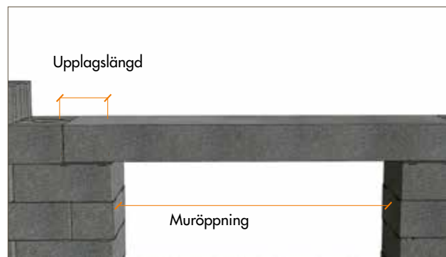
Bild 3.5 Upplag av LECA balk.
