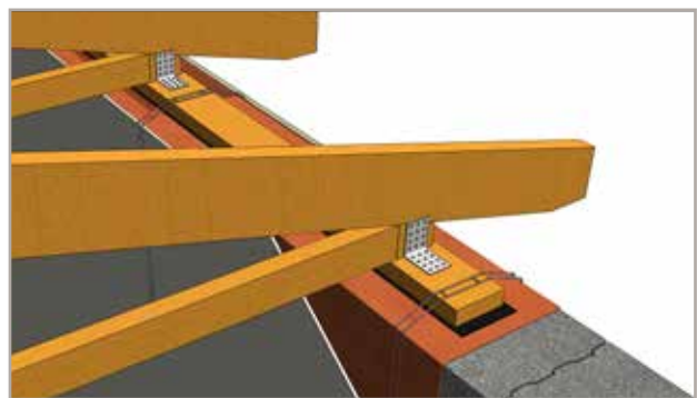
Bild 3.6 Vindförankring med bistål eller vajernät.
