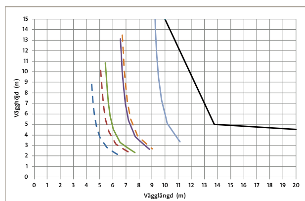
Diagram 3.6 Maximal väggstorlek för LECA block 250 med 1,2 kN/m 2 vindlast och upplag A.
