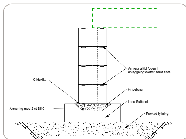
Bild 2.2 Murad grundsula, ritning L 1-301.
