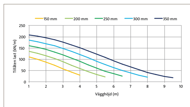
Diagram 3.3 Tillåten vertikal last vid icke centrerad last (50 mm från ytterkant).
