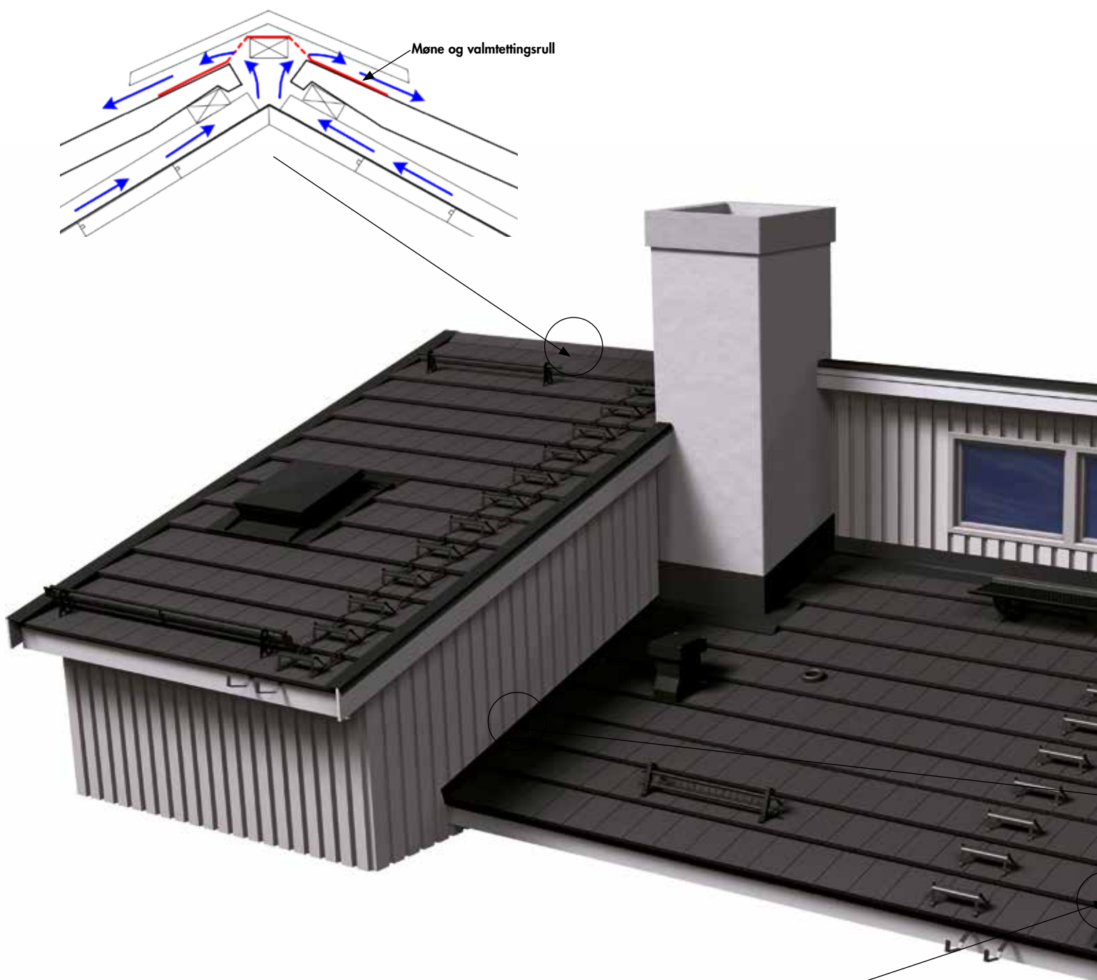
Bilde 4: Vindski, montering av skjult avrenningsbeslag.
