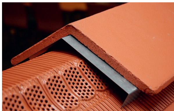
Nockbygels montering
